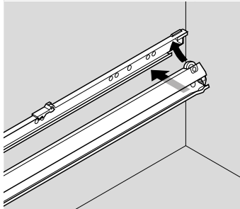
Inhangen en vergrendelen van het middenprofiel 430E
