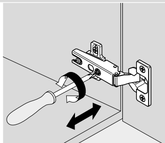
Zijdelingse verstelling
