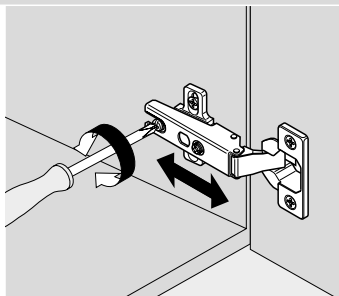
Diepteverstelling
