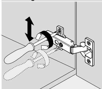
Hoogteverstelling
